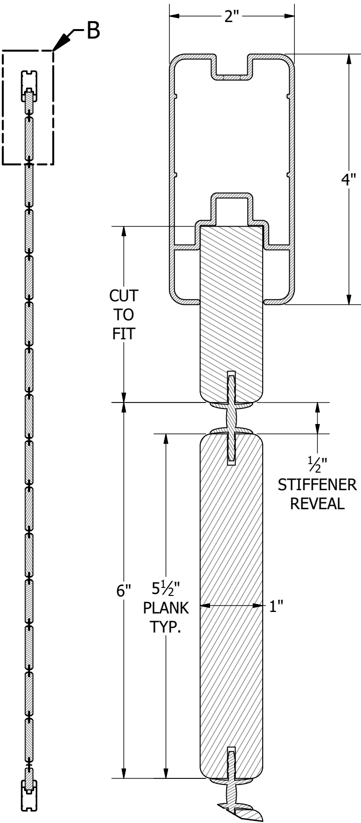
SECTION A-A
